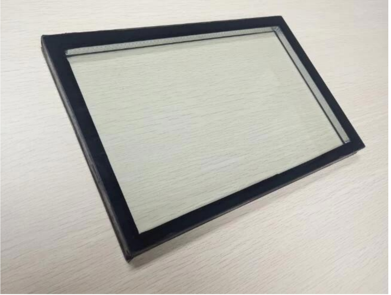
الزجاج المعزول الصين مستودع e ملليمتر منخفضة 5 + 12a + 5
