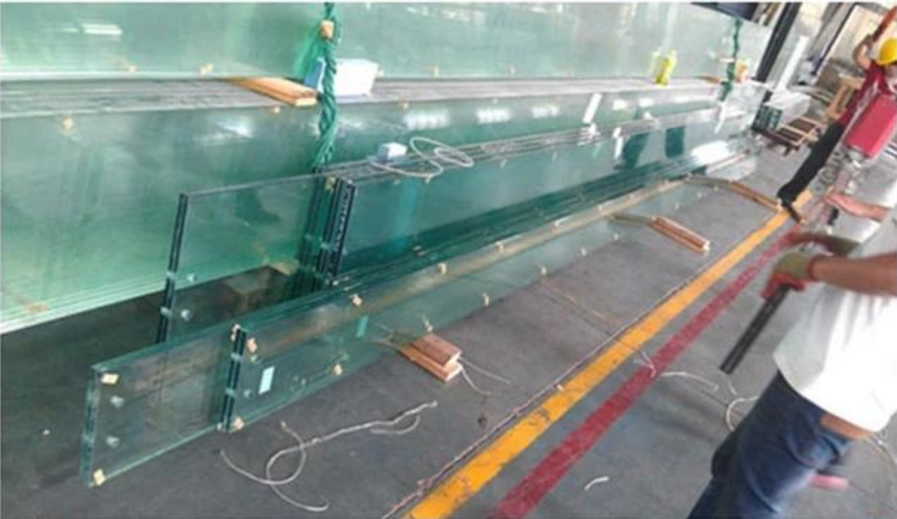
Differ Design-Glasrippen-Stützstruktur:
