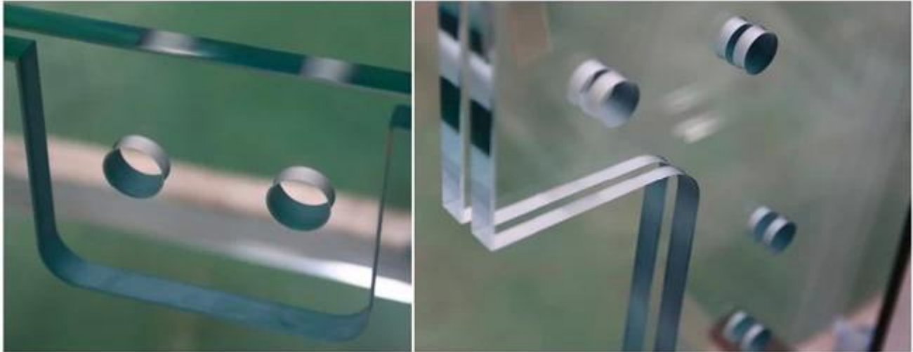
Ausgeglichenes lamelliertes Glas mit Ausschnitte und Bohrungen
