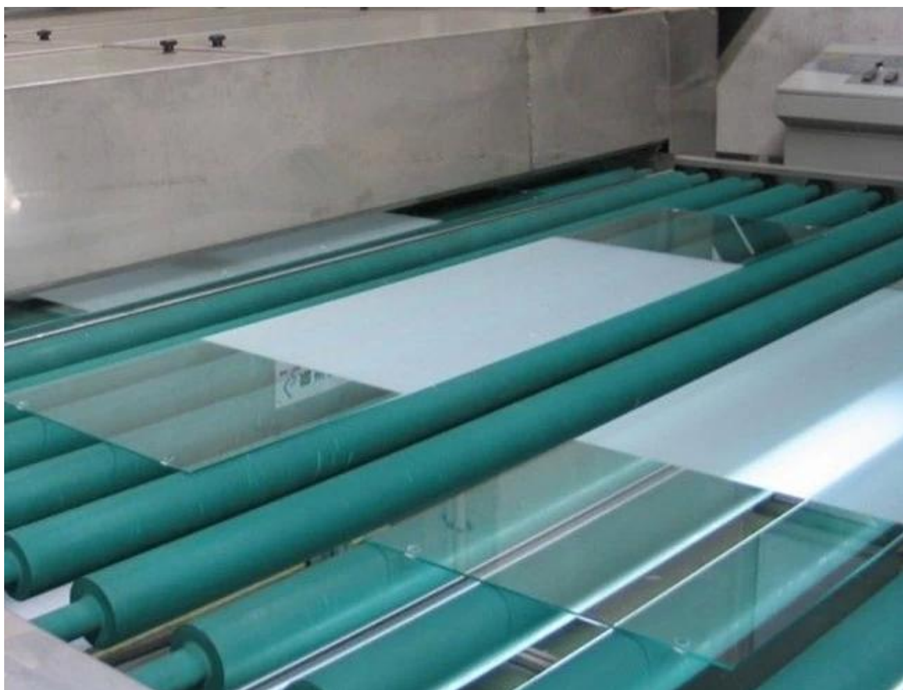
Production ligne de verre dépoli acide
